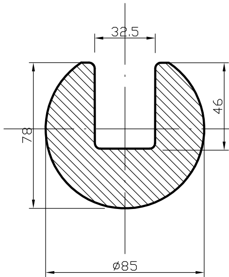
B-B
